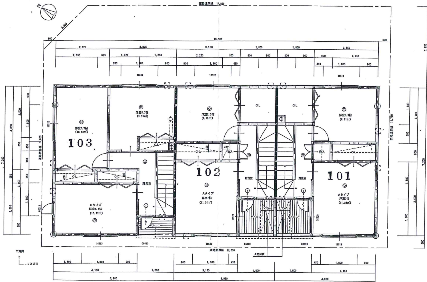
2階 平面詳細図 5:1/50
