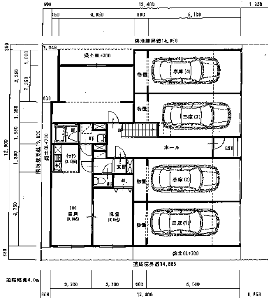
配置図・地階平面図1/100
