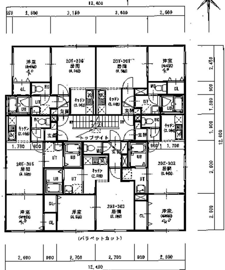
1F・2F平面図1/100
