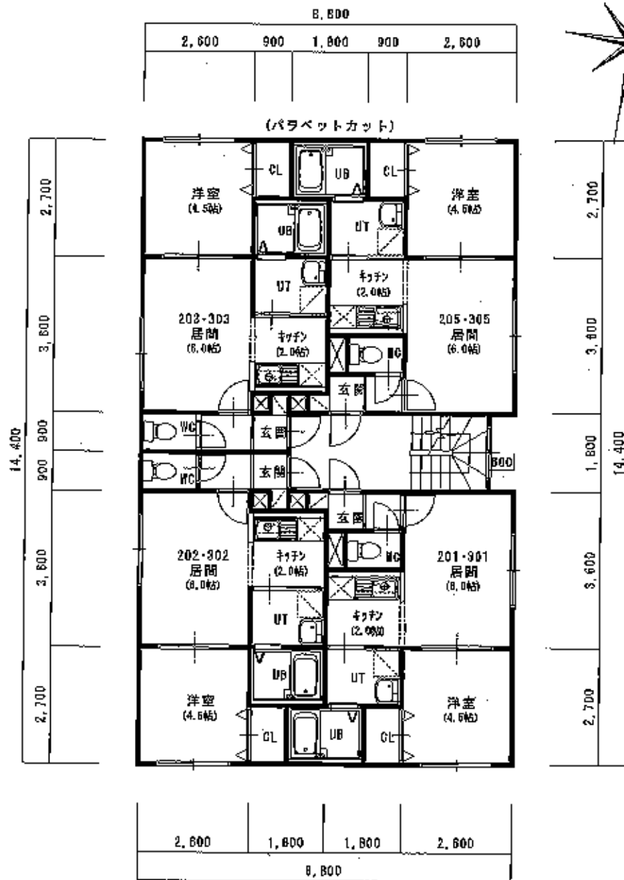
1F・2F平面図1/100
