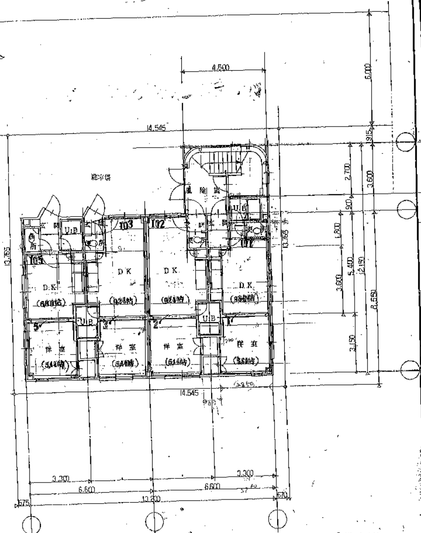
1階平面図
