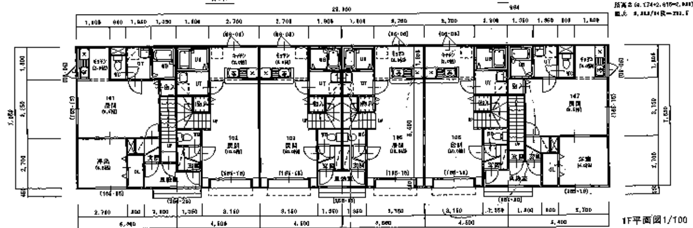
(仮称)箱館2-1マンション計画案<D案>
