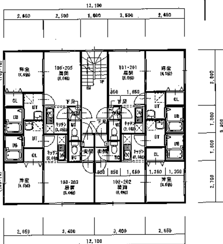
1F・2F平面図1/100
