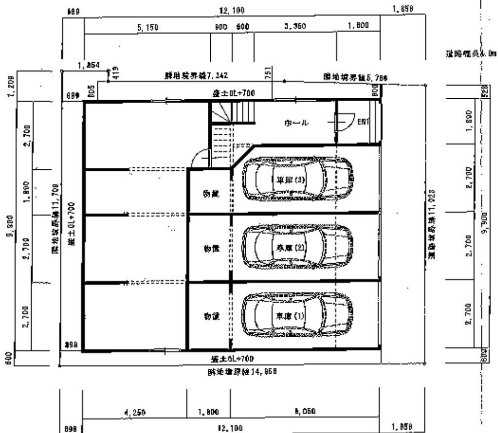
配置図・地階平面図1/100
