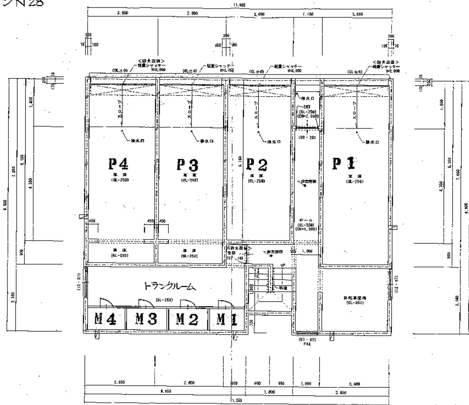
地階平面詳細図 1/50
