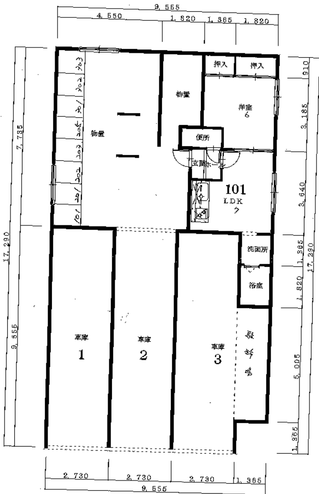
1階平面図
