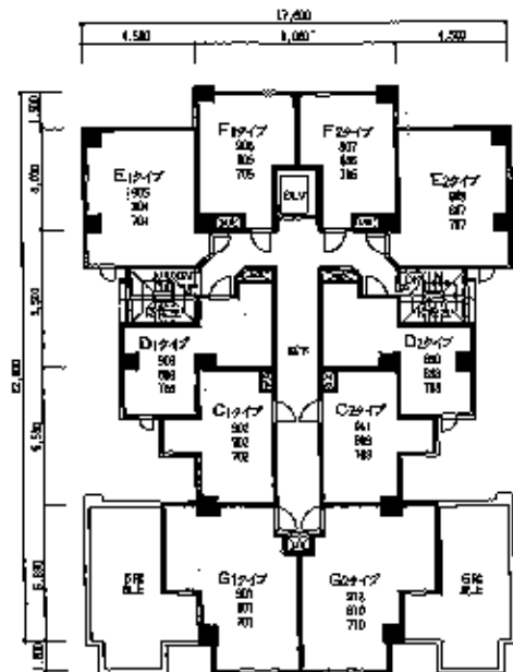
7~9階平面図
