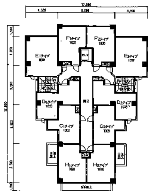
10階平面図
