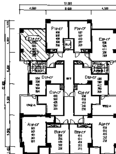
2~6階平面図
