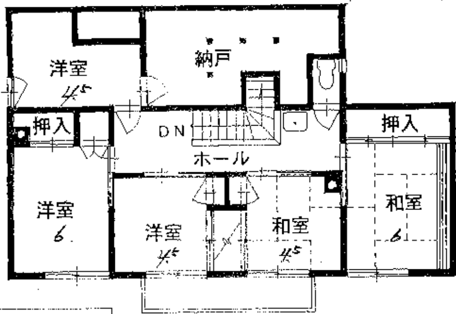
2階平面図
