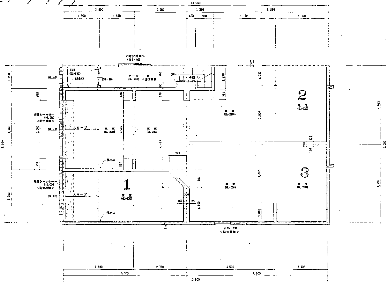
地階平面詳細図 1/50
