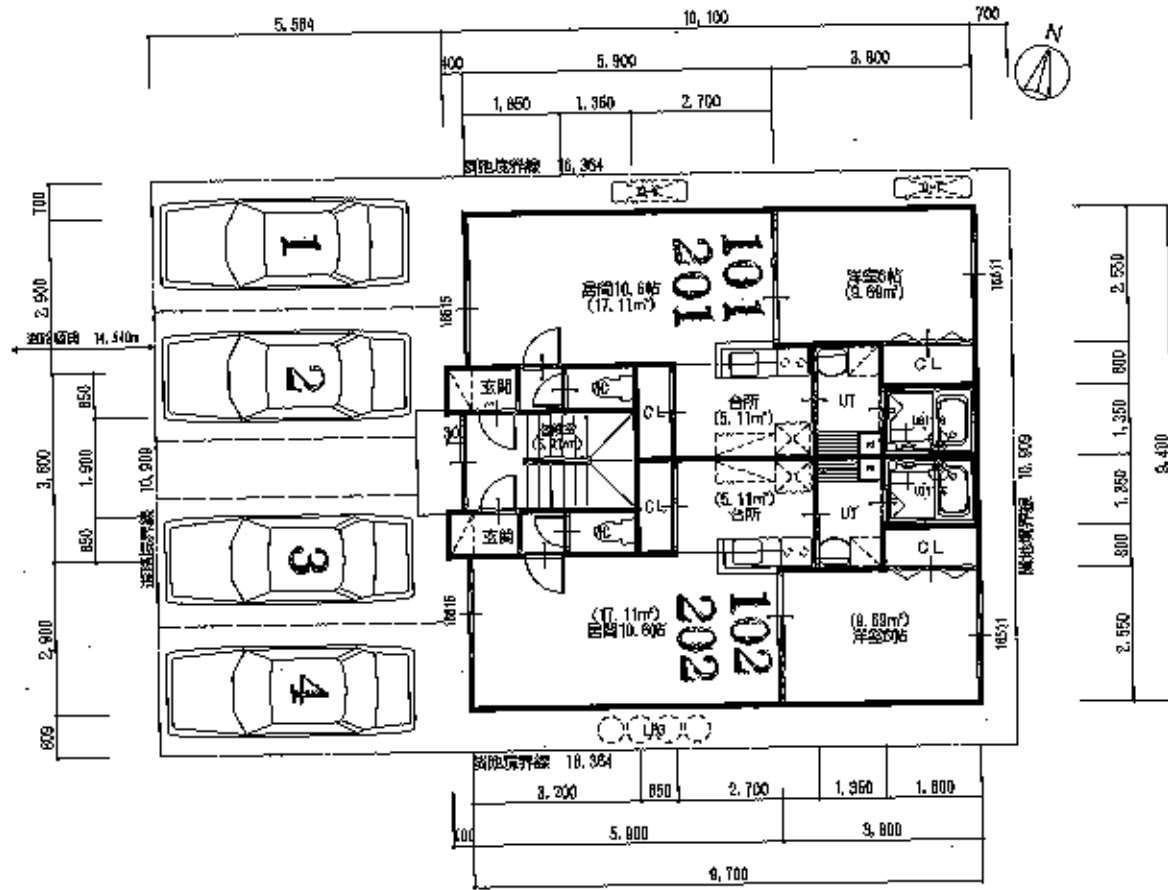
1-2階 平面図 8: 6/100
