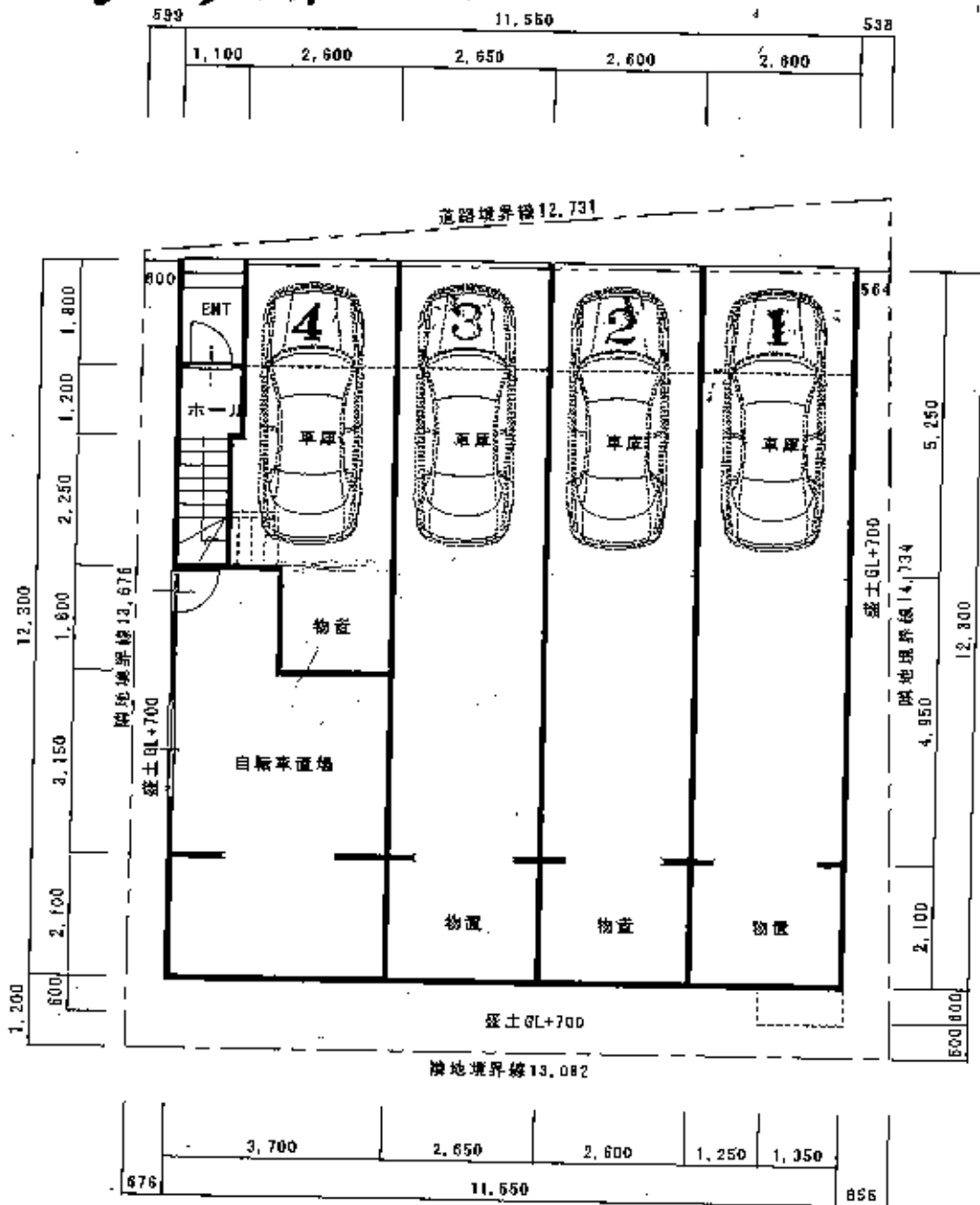
配置図・地階平面図 1/100
