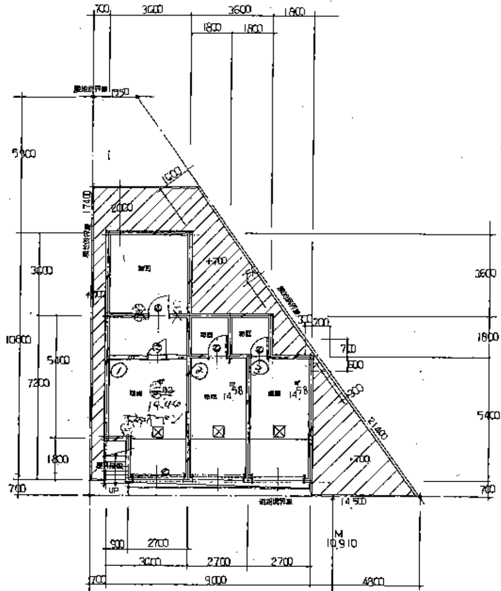
B1階平面図 S=1/100
