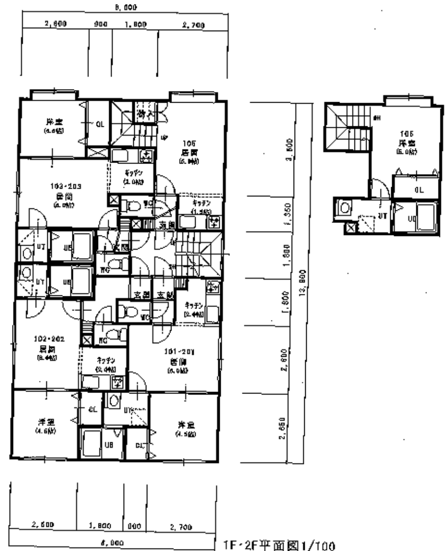
1F・2F平面図1/100
