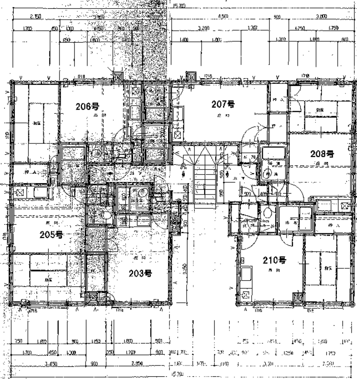
2F平面図 1/500
