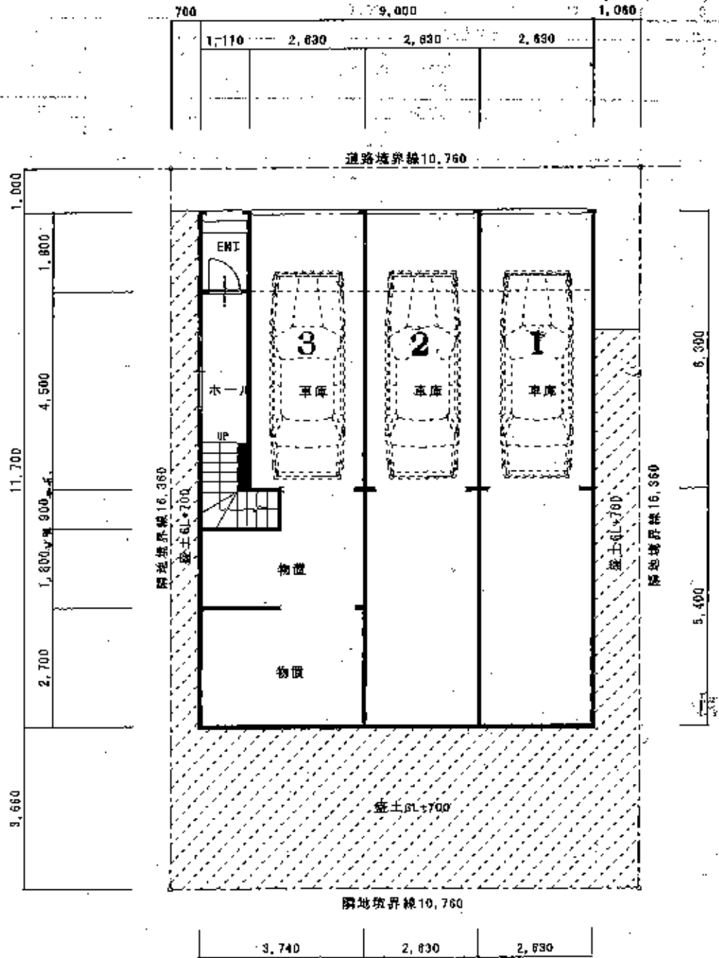
配置図・地階平面図1/100
