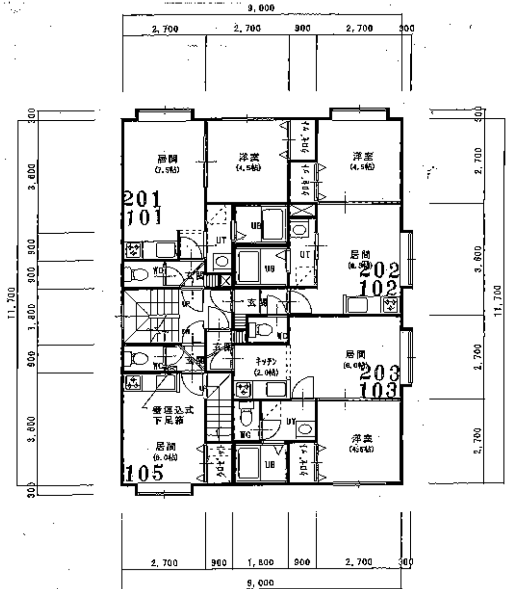
1F・2F平面図1/100
