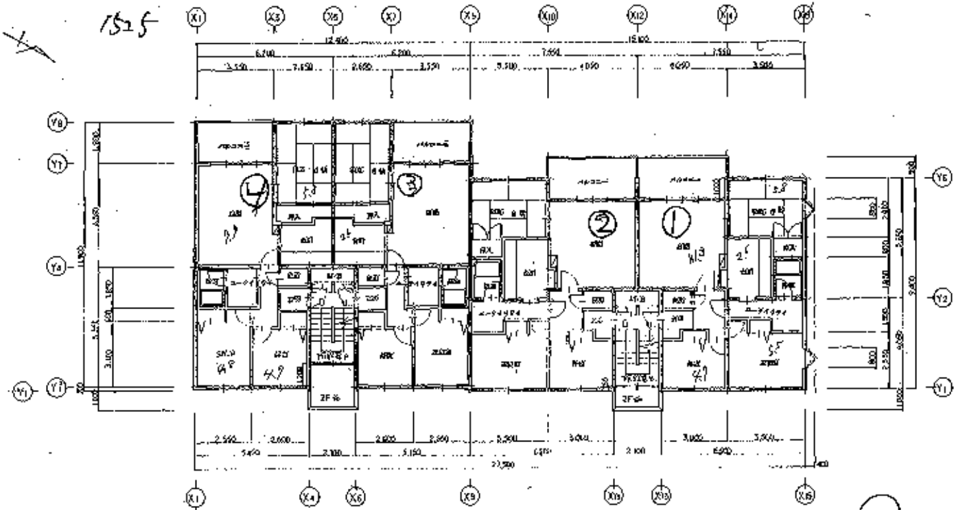
2F 階平面図 3F
