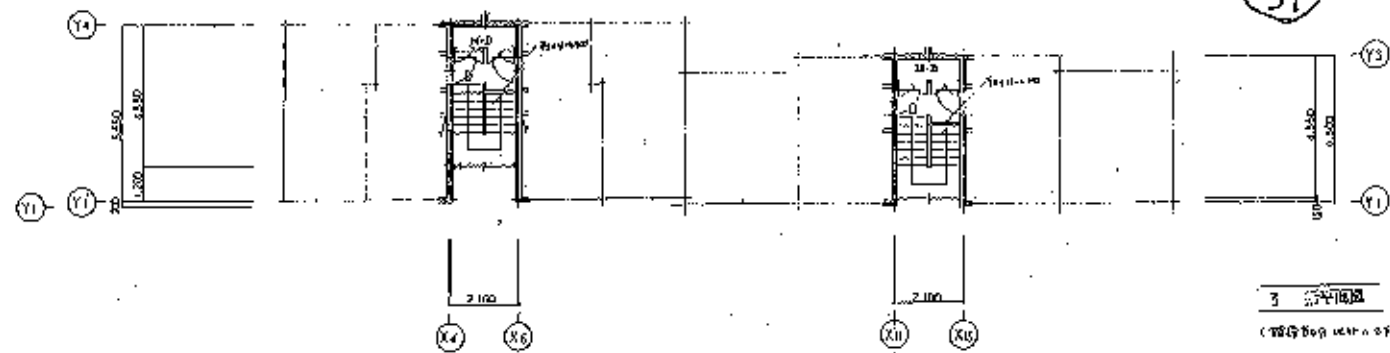
2F 階平面図 3F
