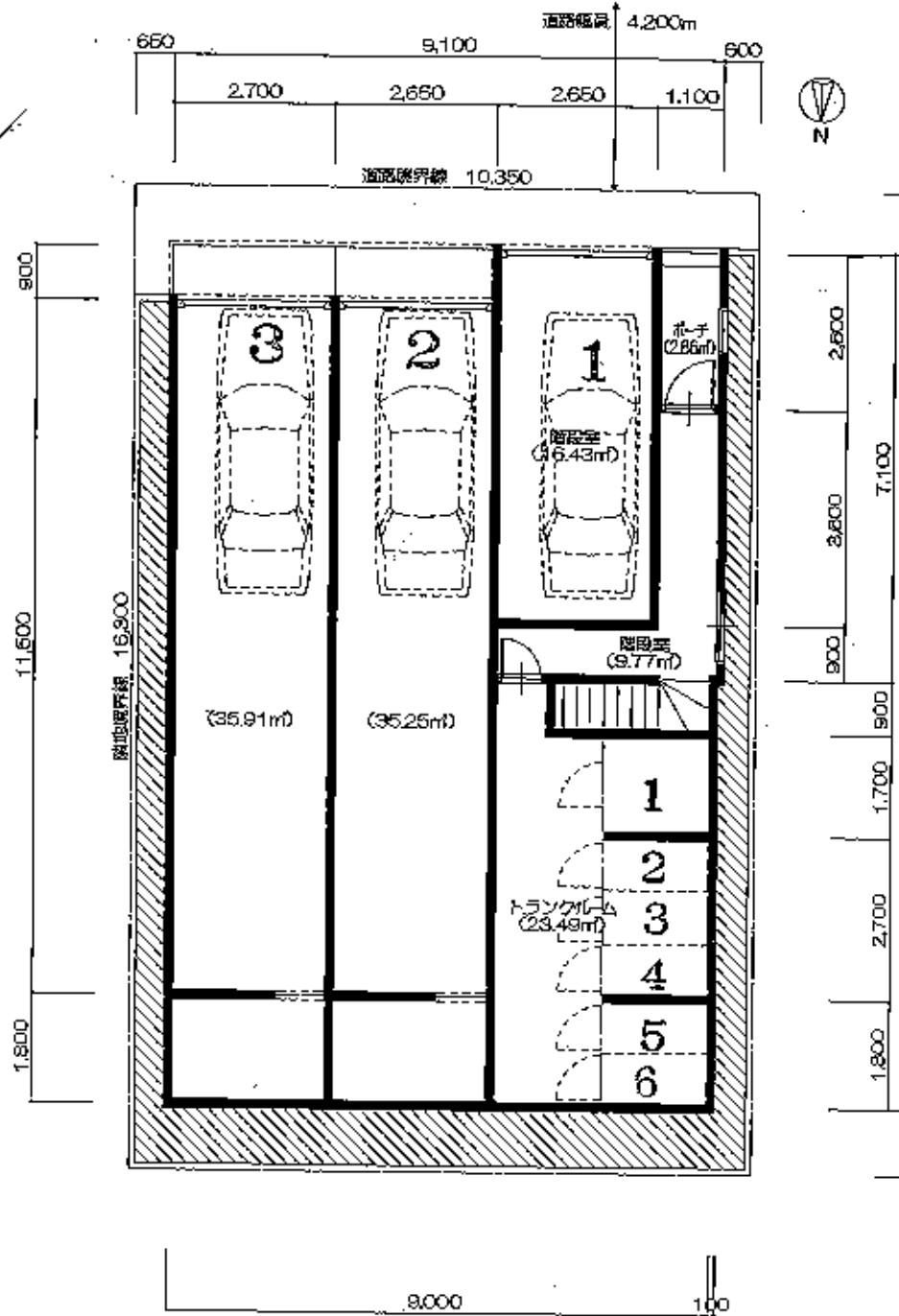
地下1階 平面図 S1/100
