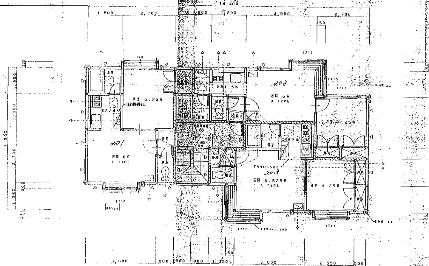
2階平面図 1/50
