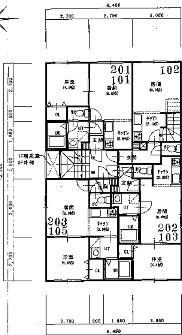
1F・2F平面図1/100
