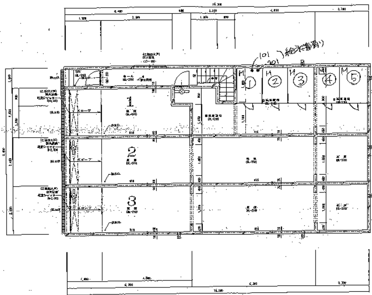
地階平面図 1/50
