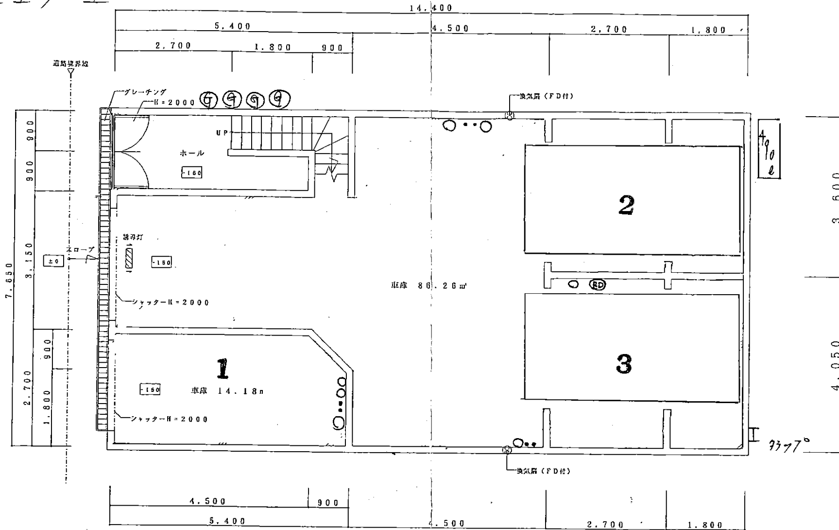
地階平面図 1 / 50
