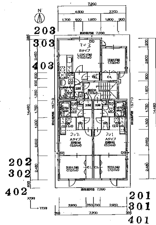
2-4階 平面図 S1/100
