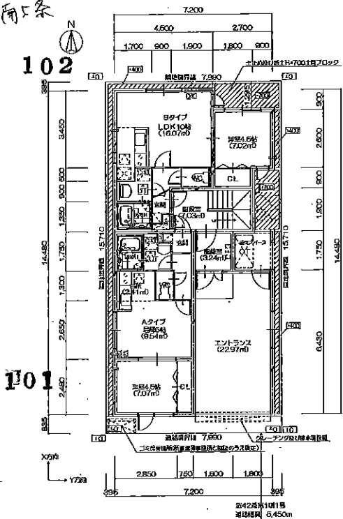
1階 平面図 S1/100
