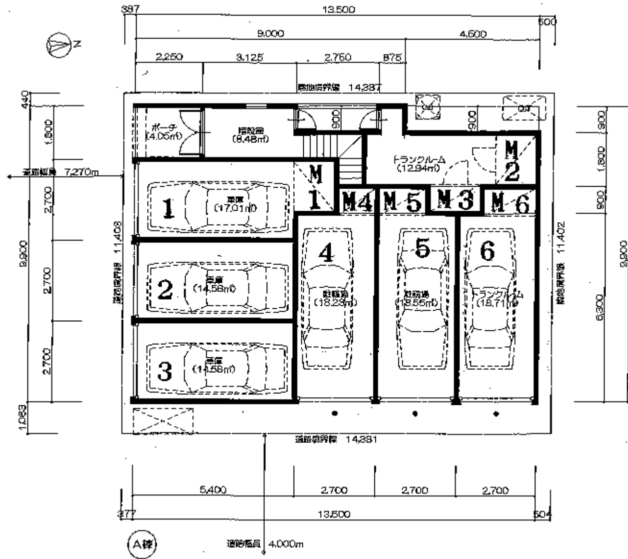
地下1階 平面図 S:1/120
