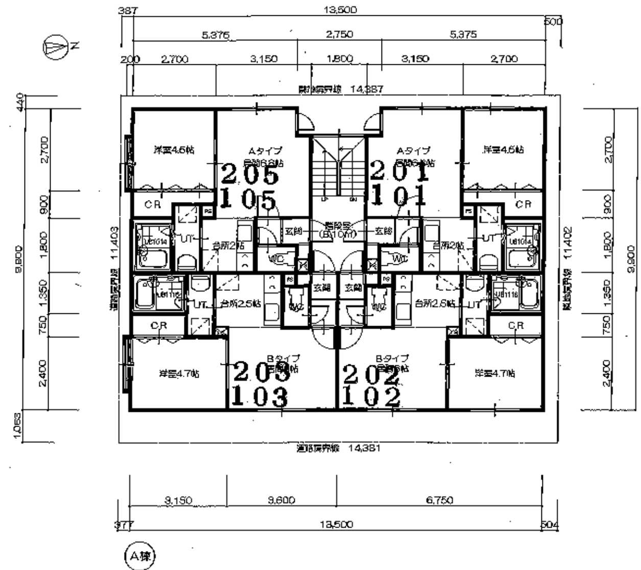
1-2階 平面図 S:1/120
