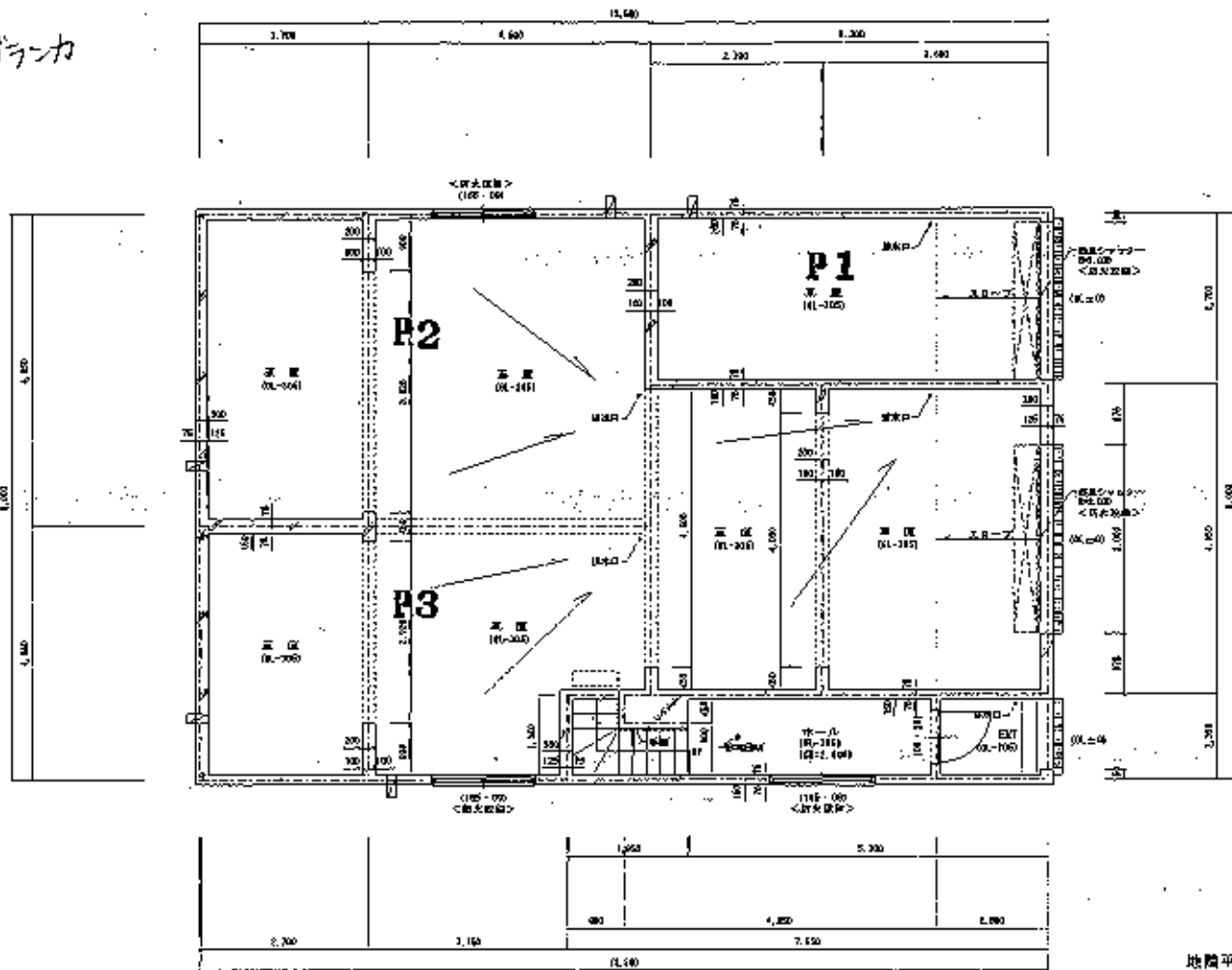
地階平面詳細図 1/50
