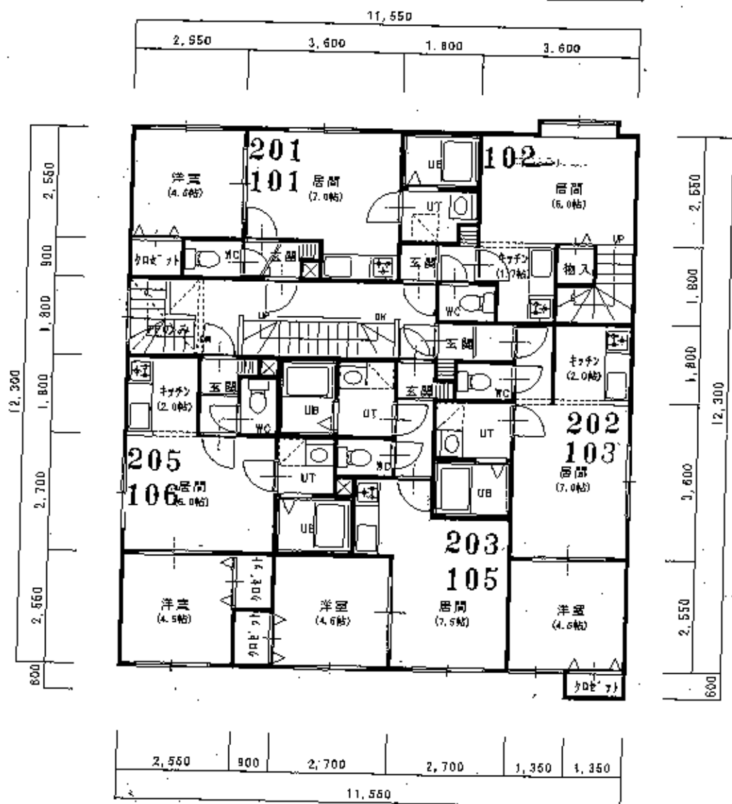
2F平面図1/100
