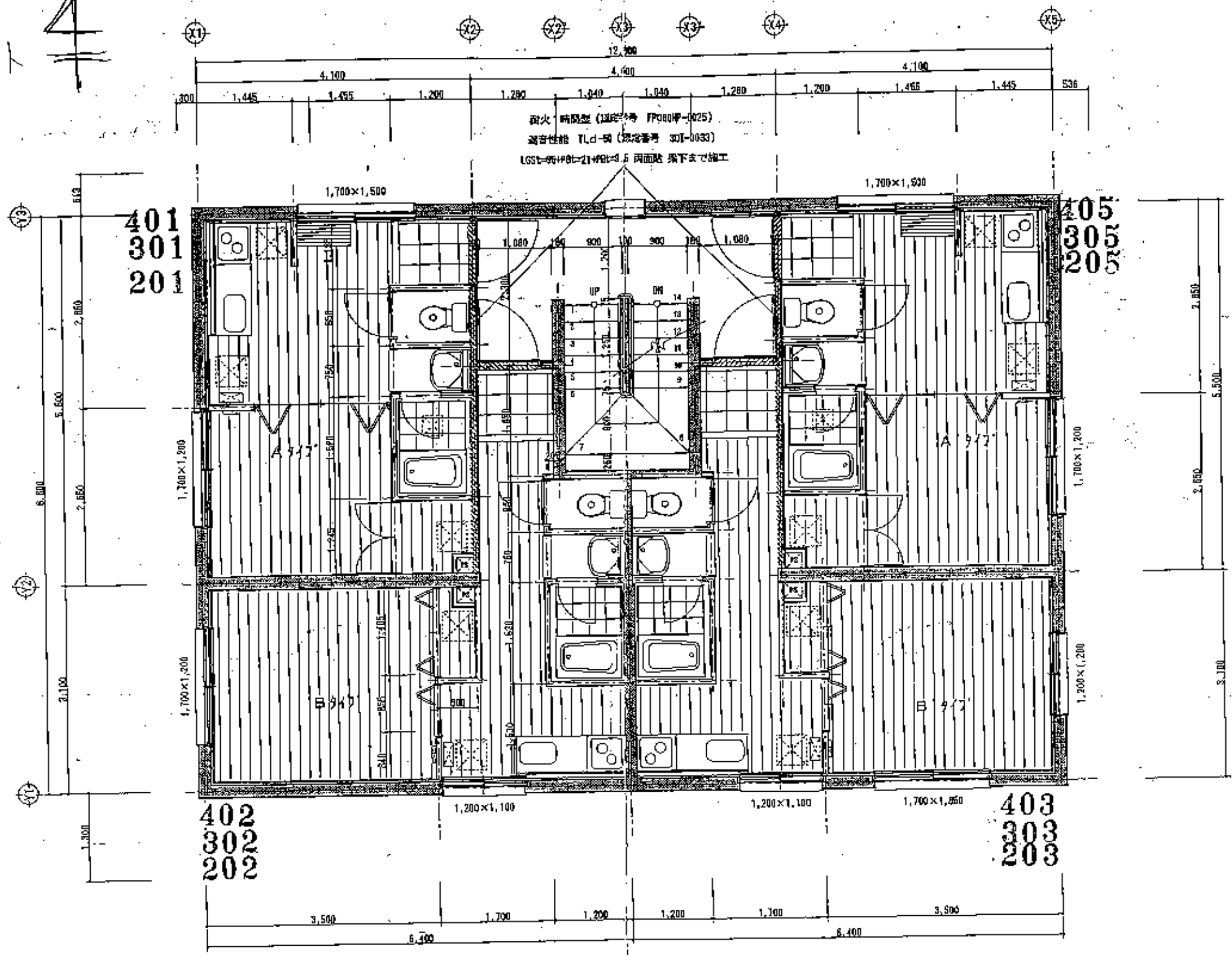
2・3階平面図
