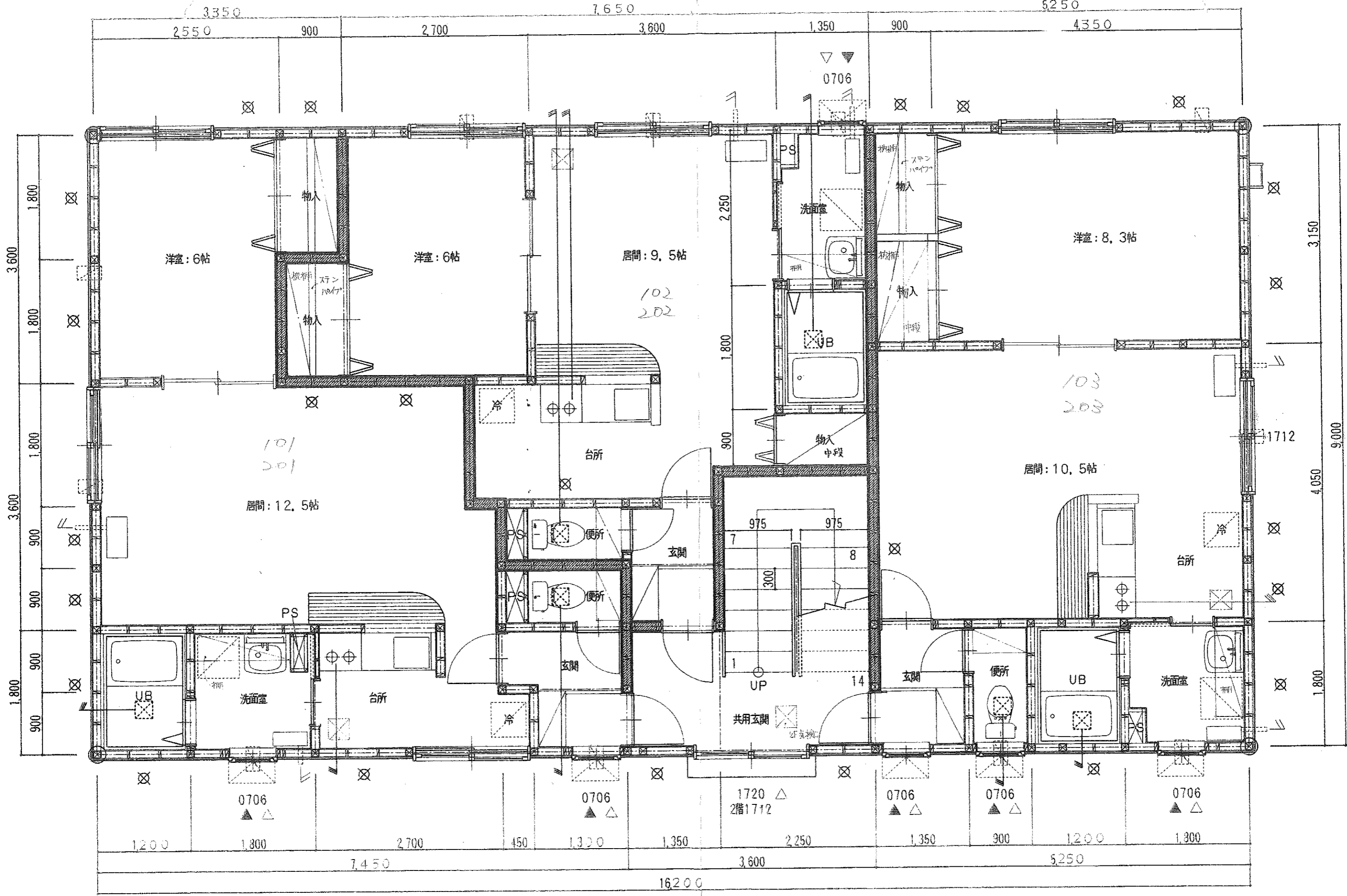
改築後1階(2階)平面図 1:50
