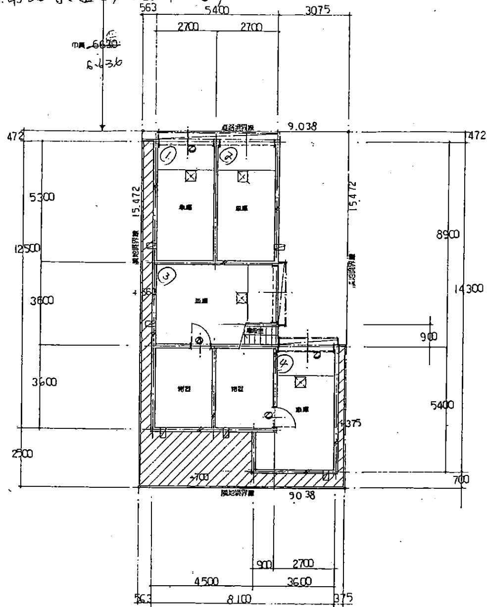
B1 階平面図 S=1/100
