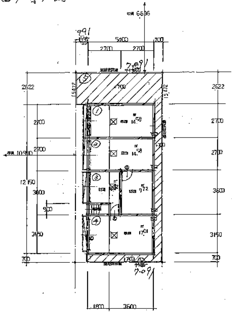
B1階平面図 S=1/100
