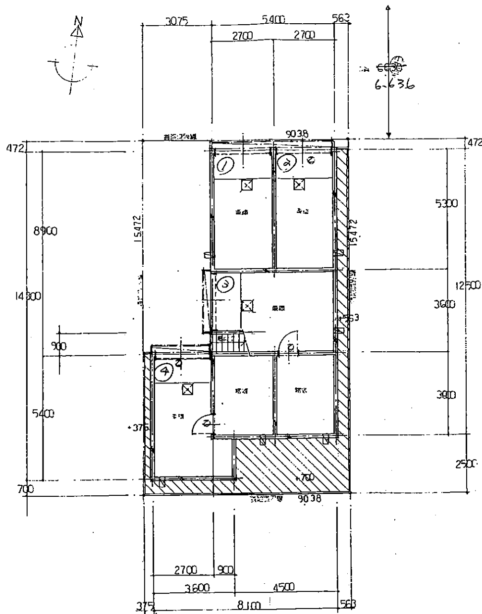
8階平面図 S=1/100
